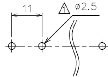
基板取付穴寸法
